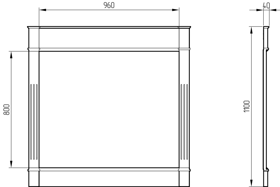
Vista posteriore/Rear view/Вид сзади
