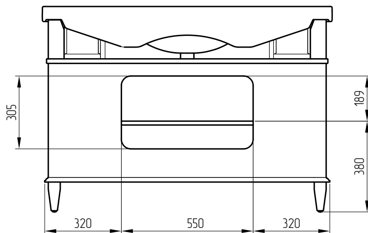
Vista posteriore/Rear view/Вид сзади
