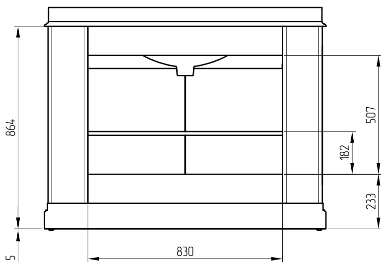
Vista posteriore/Rear view/Вид сзади
